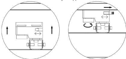
Рисунок 9. Крепление на шинпроводе.
